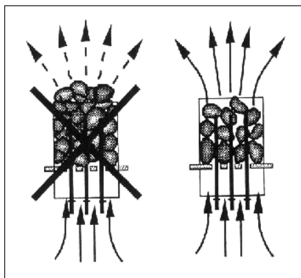
Figure 1. Piling of the sauna rocks Figure 1. Mise en place des pierres du poêle
